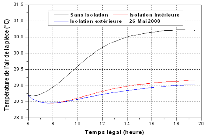
Fig.(4.3): Température de l'air intérieur de la pièce
