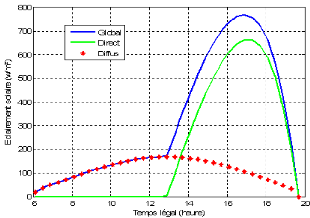
Fig.(3.7): Eclairement solaire incident sur le mur Ouest
