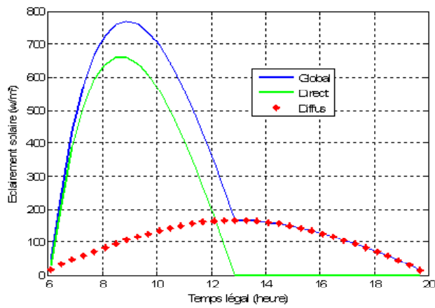
Fig.(3.6): Eclairement solaire incident sur le mur Est
