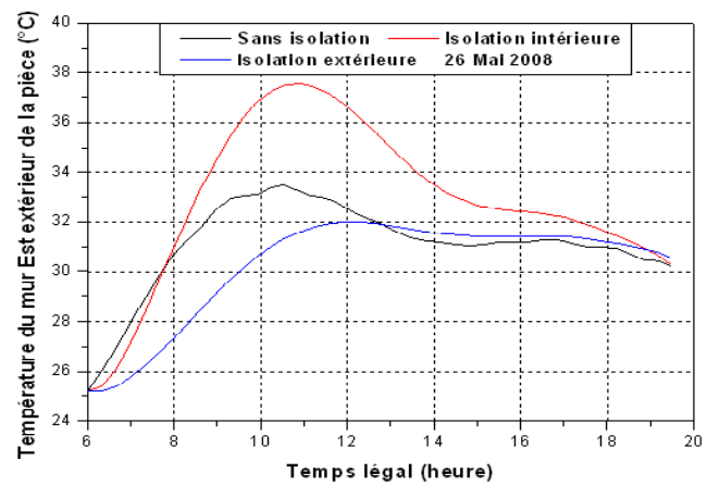
Fig.(4.4): Température de la paroi extérieure du mur Est de la pièce
