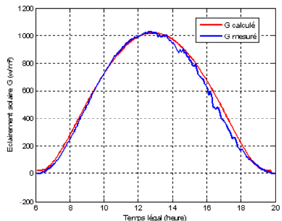
Fig.(3.4): Éclairément global sur un plan incliné par 32^\circ , 26 / 05 / 2008.
