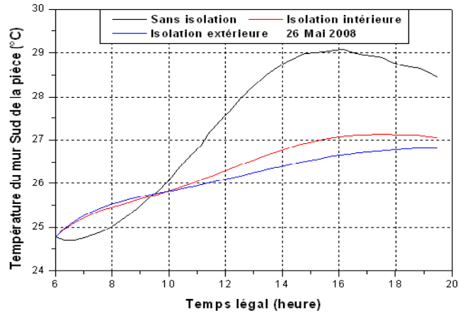
Fig.(4.2): Température de la paroi intérieure du mur Sud de la pièce
