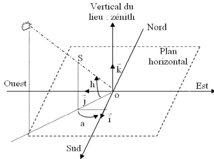
Fig.(3.2): Repère horizontal
