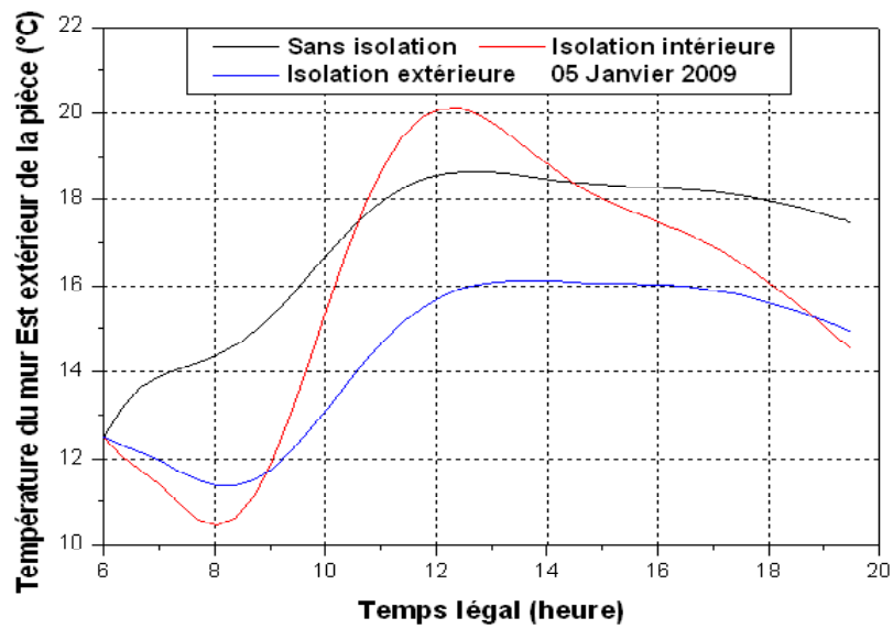
Fig.(4.7): Température de la paroi extérieure du murd Est de la pièce
