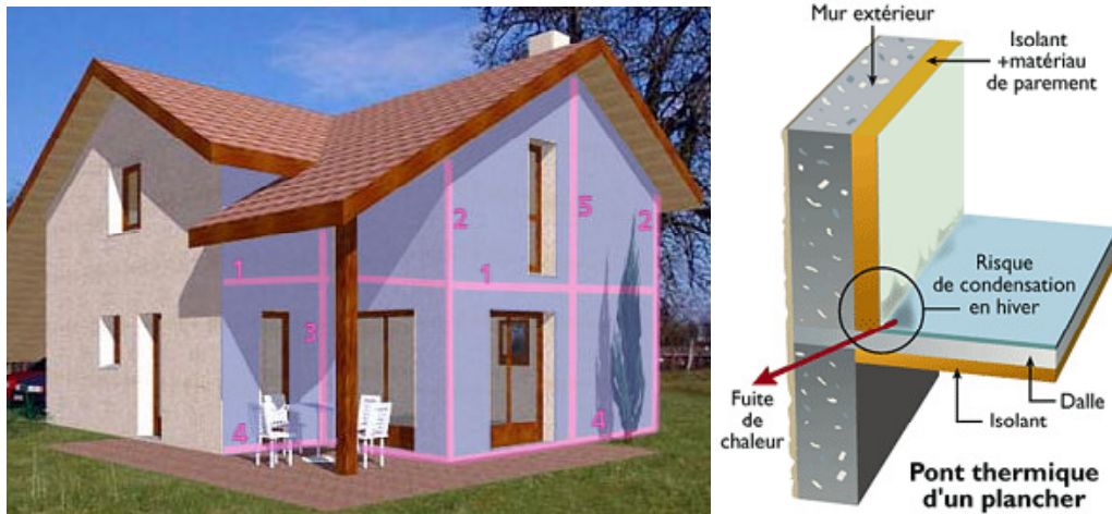
Fig.(4.1): Illustration des ponts thermiques de liaison.
