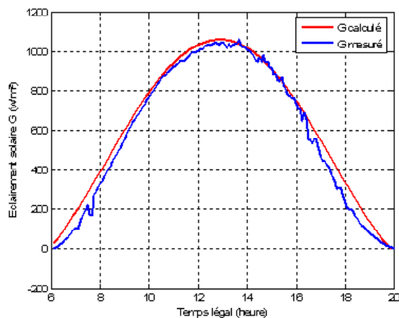
Fig.(3.3): Éclairément global sur un plan horizontal, 26 / 05 / 2008.
