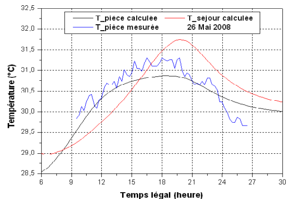
Fig.(3.9): Température de la pièce et de la salle de séjour, 26 Mai 2008.
