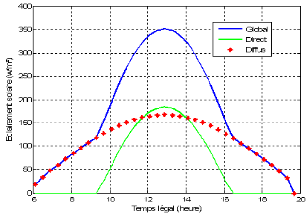
Fig.(3.5): Eclairement solaire incident sur le mur Sud
