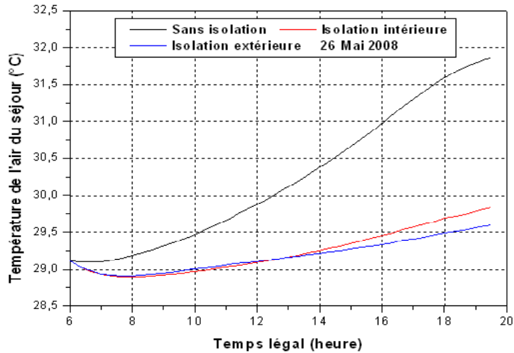
Fig.(4.5): Température de l'air intérieur de la salle du séjour
