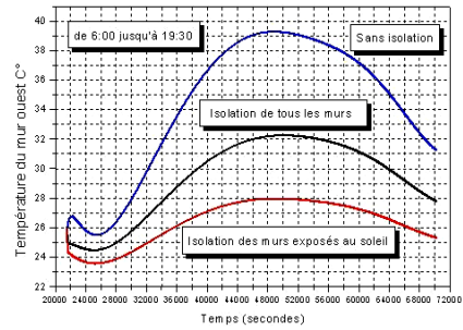
Fig. 10: Température du mur Ouest
