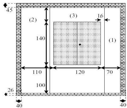
Fig. 2: Mur Sud
