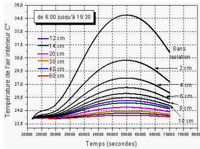
Fig. 29: Influence de l'épaisseur de l'isolant sur la température de l'air intérieure de la pièce
