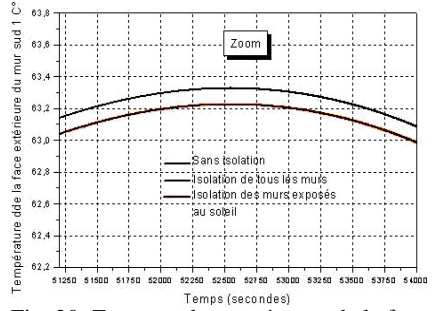
Fig. 20: Zoom sur la température de la face extérieure du mur Sud 1
