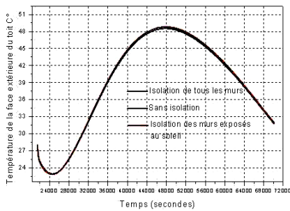
Fig. 15: Température de la face extérieure du toit
