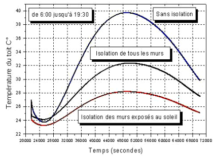
Fig. 14: Température du toit
