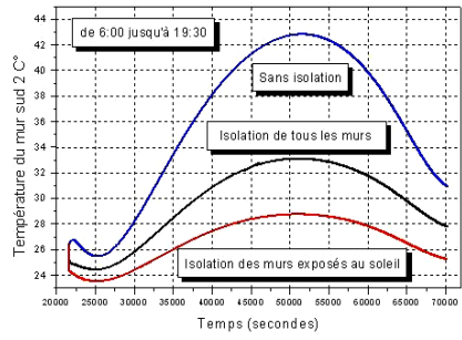
Fig. 22: Température du mur Sud 2
