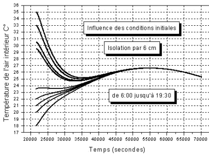
Fig. 30: Influence des conditions initiales sur la température de l'air intérieure de la pièce
