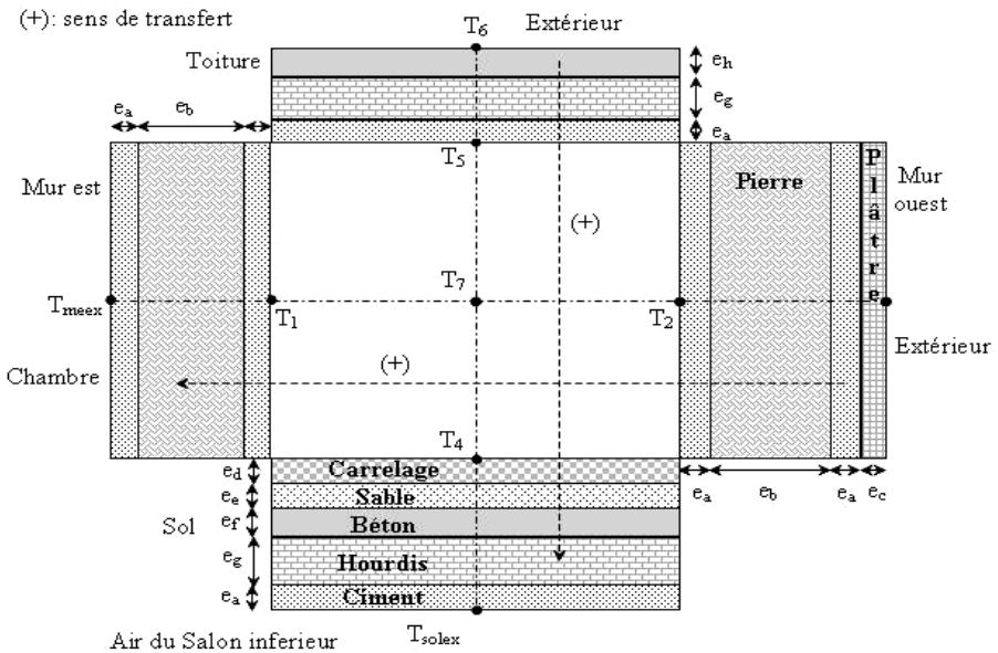
Fig. 4: Coupe longitudinale
