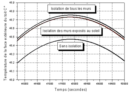
Fig. 16: Température de la face extérieure du toit
