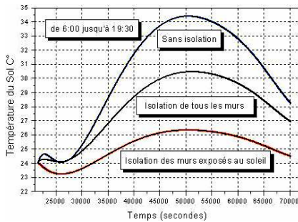
Fig. 13: Température du sol
